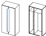
379.01 Шкаф 2 дв.(с зеркалом) 1000x594x2172 379.0101 К-т полок д/шир. секции (2шт.) 379.0202 К-т полок д/узкой секции (2шт.)
