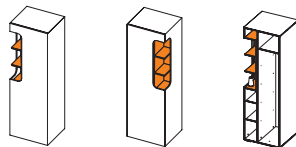
379.02 Шкаф 1 дв. (левый/правый) определяется по стеллажу 600x594x2172 379.0202 К-т полок (2шт.)
